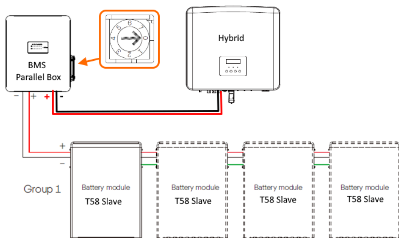
התקנת מערך בודד
