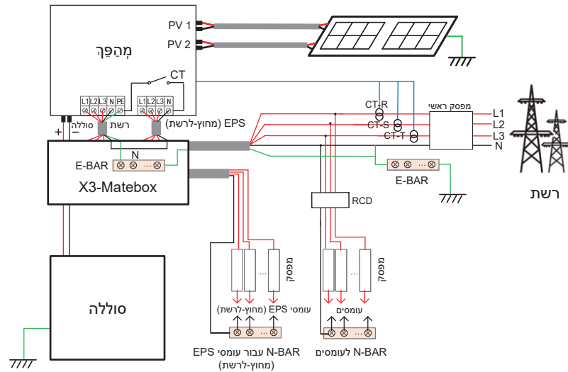
תרשים ד': קו N וקו PE יחד, כל ערכת EPS של חיבור עומס (מחוץ-לרשת); (ישיבאוסטרליה)
