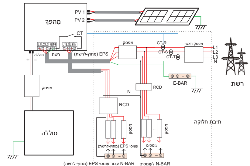
תרשים ג': קו N וקו PE יחד, מהפכים מסדרת (ישם באוסטרליה)
