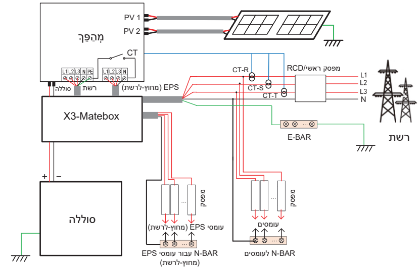
תרשים ג': קו N וקו PE יחד, מהפכים מסדרת (ישם באוסטרליה)
